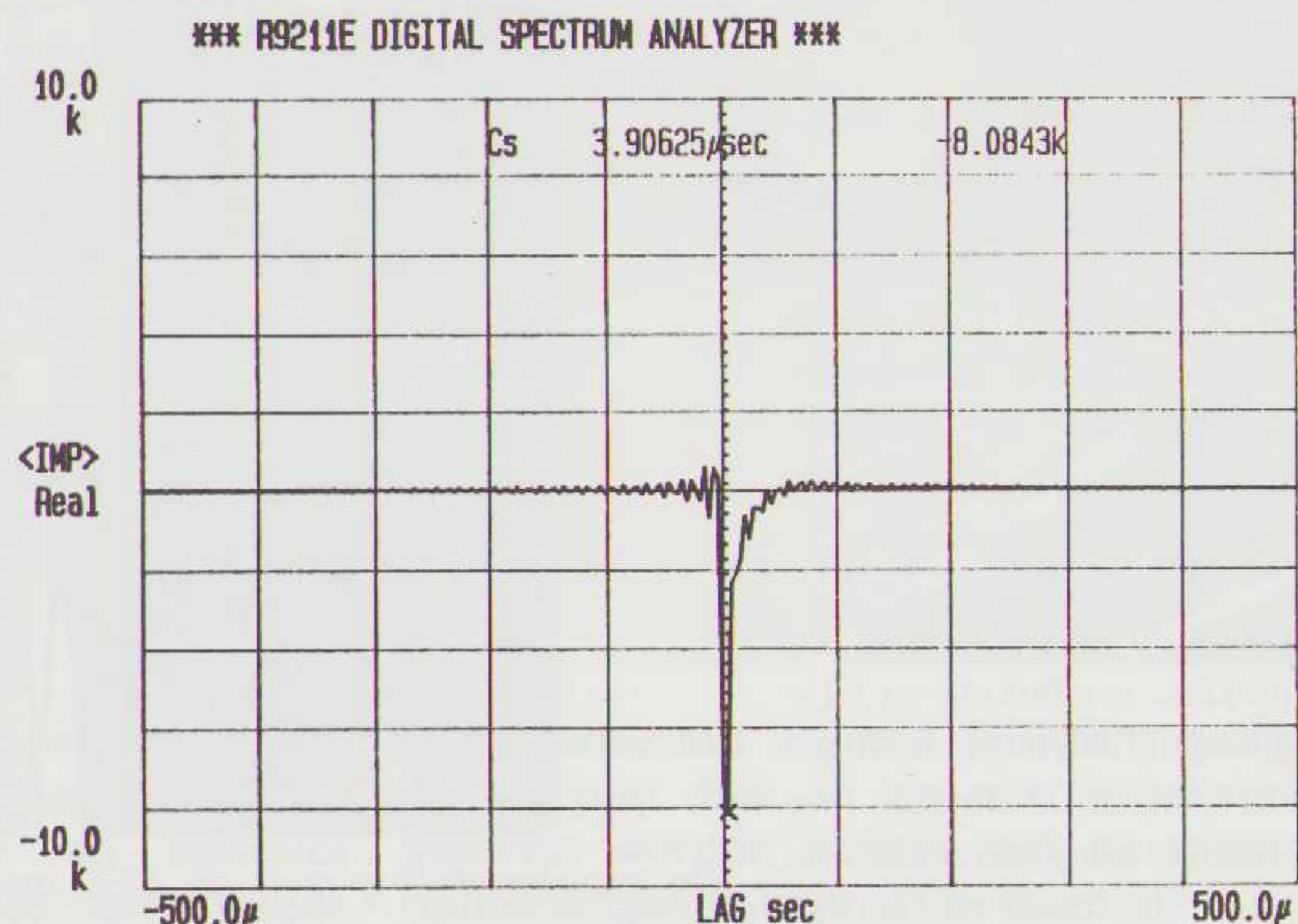
De impulsrespons van de A-80 eindversterker
